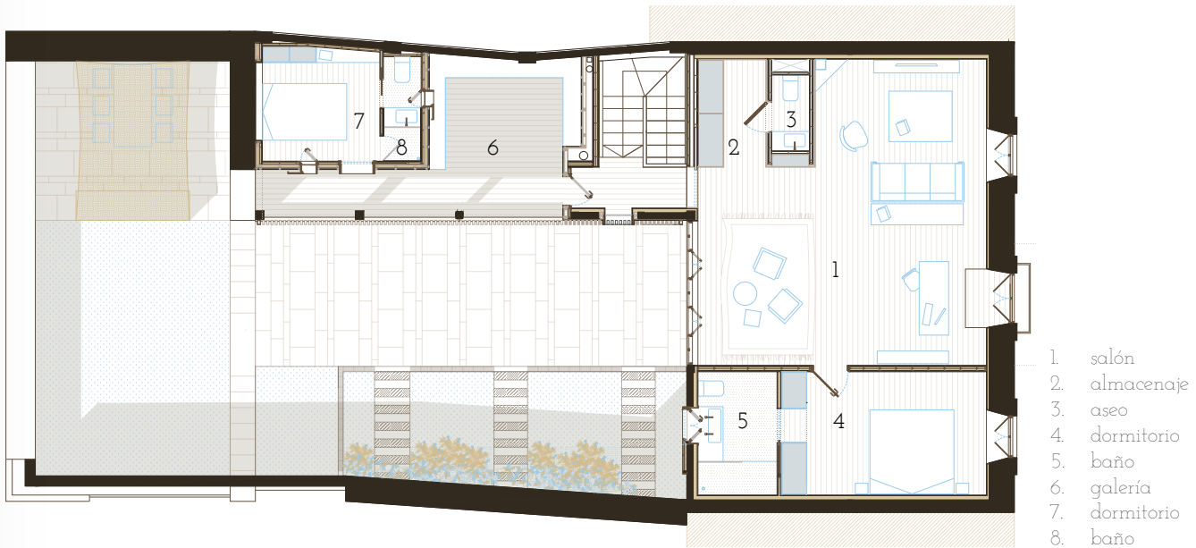
planta primera
